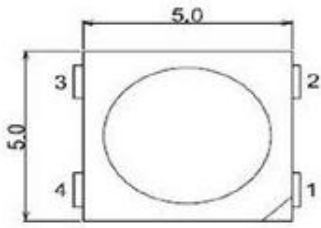
封装尺寸 Package Dimensions
